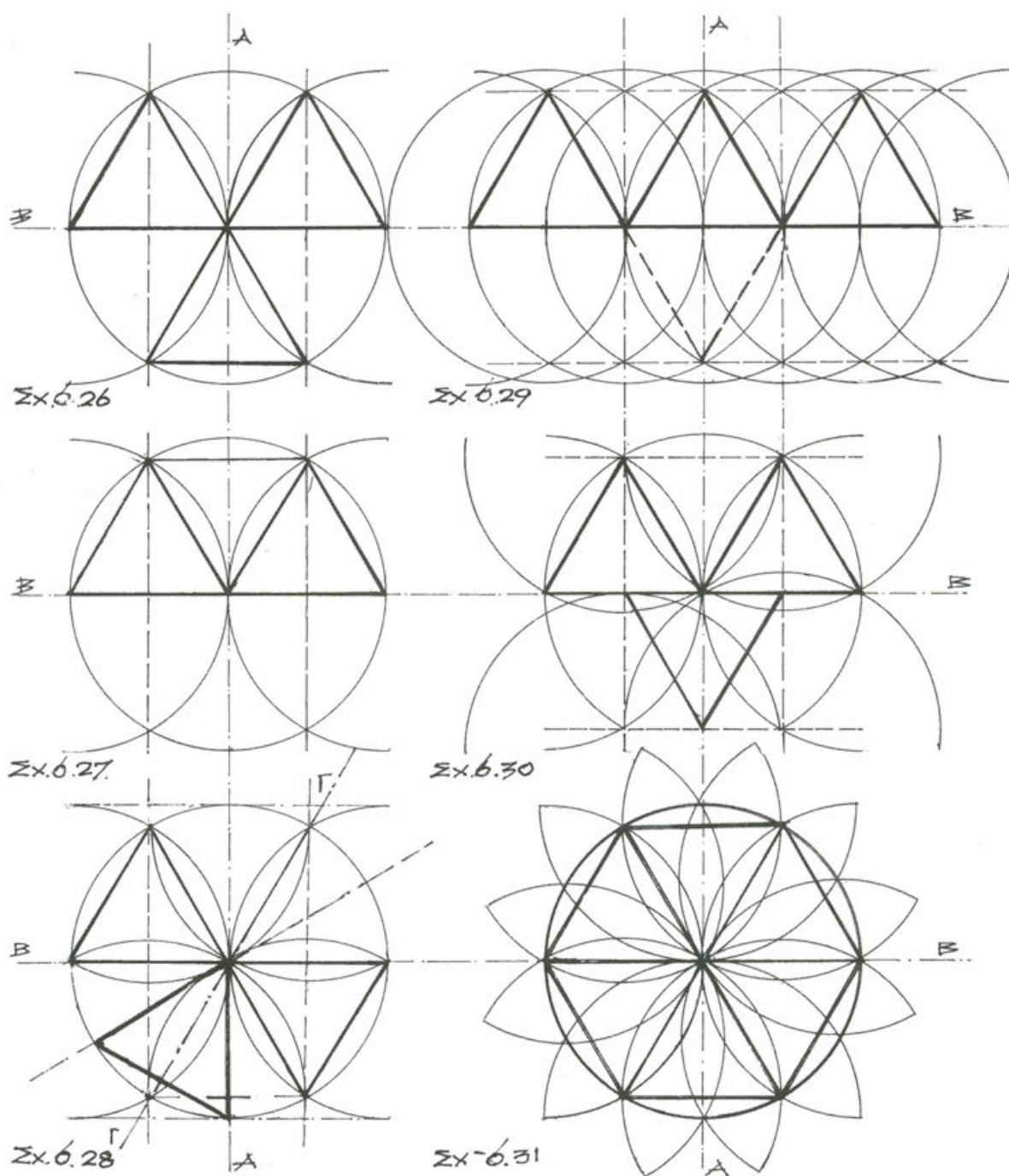
Σχ. 6.26 - 6.31 Συμμετρικές διατάξεις τριών ισοπλευρων τριγώνων σε παραλλαγές
