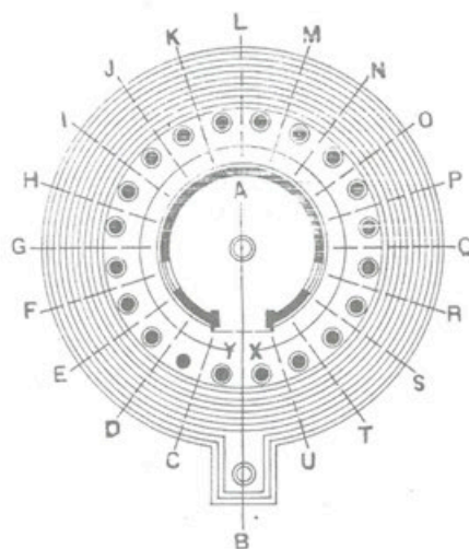
Εικ.6.19 Στο αρχαίο ημικυκλικό θέατρο (10α) συναντάμε την περίπτωση της σύγκλισης πολλών αξόνων προς ένα κεντρικό σημείο παρατήρησης σε συμμετρική ακτινική διάταξη. Η ακτινική διάταξη έχει εφαρμοστεί και στο ναό της Αφροδίτης στη Ρώμη (10β).
