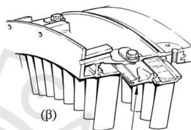
(β) Στεφάνη στηρίξεως των περυγίων επί του εξωτερικού κελύφους
