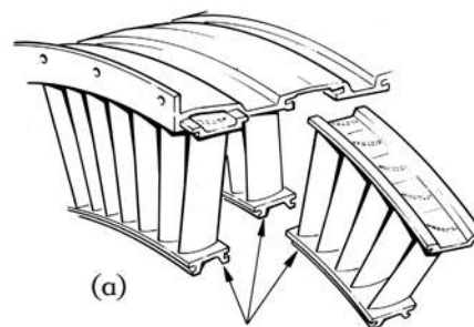
(α) Περύγια σιάτορα με κέλυφος (στεφάνη)
