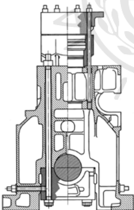
Σχ. 5.2ιβ Μορφή και τοποθέτηση συνδετών σε τετράχρονη μεσόστροφη εν σειρά πετρελαιομηχανή.
