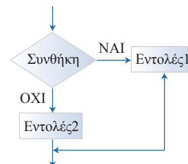
Εικόνα 4-4. Διάγραμμα ροής της σύνθετης επιλογής
