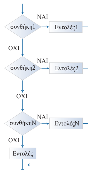
Εικόνα 4-5. Διάγραμμα ροής της πολλαπλής επιλογής
