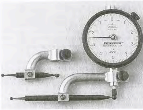
Σχήμα 3.2.3α. Μετρητικό ρολόι με τα εξαρτήματά του – Χρήση του μετρητικού ρολογιού για τον έλεγχο της κυλινδρικότητας άξονα
