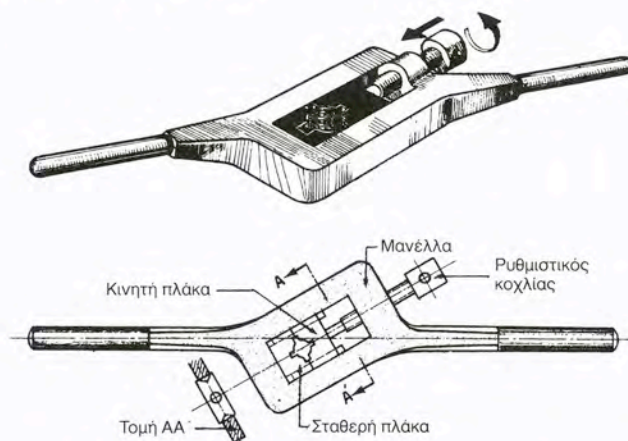
Σχήμα 4.16ζ. Διμερής ή διαιρούμενος βιδολόγος
