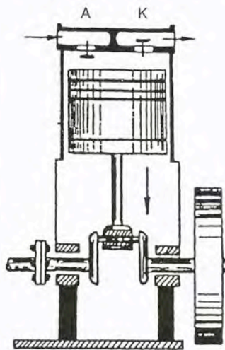
Σχήμα 16.2.1 α. Τομή εμβολοφόρου παλινδρομικού αεροσυμπιεστή Α: Αναρρόφηση Κ: Κατάθλιψη
