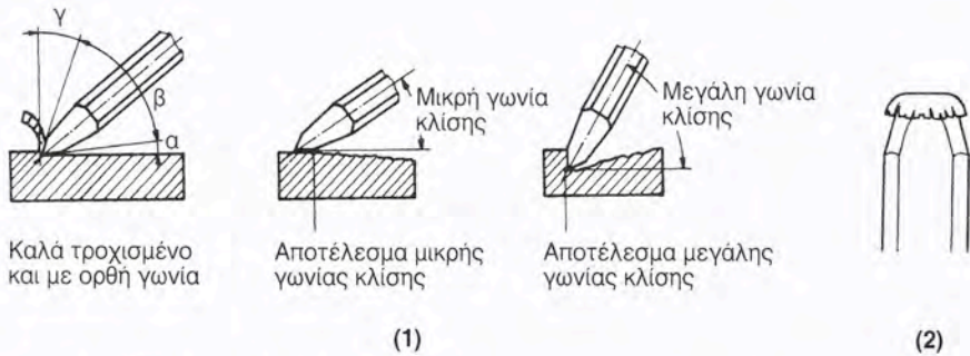
Σχήμα 4.8γ -1. Ορθή κλίση κοπιδιού κατά το κοπίδισμα -2. Κεφάλωμα
