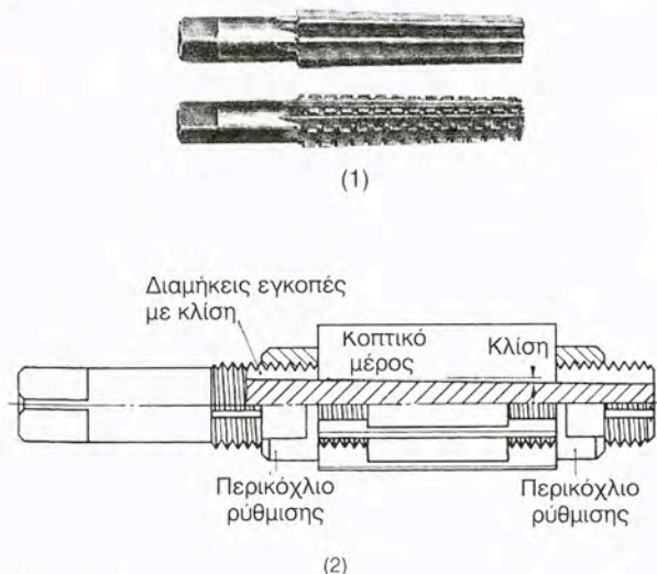
Σχήμα 4.158 -1. Κωνικά γλύφανα χειριού
