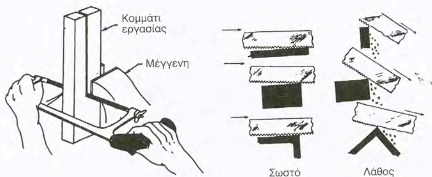
Σχήμα 4.9ε. Σωστή χρήση του πριονιού
