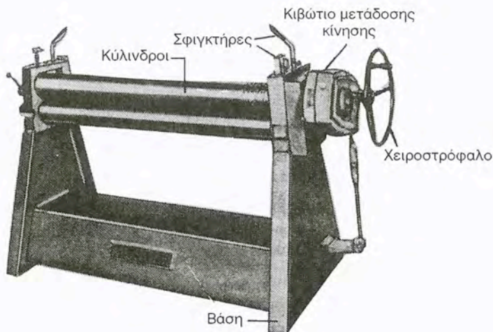
Σχήμα 6.3δ. Χειροκίνητος κυλινδροπριστής
