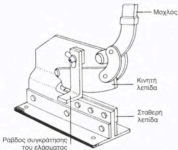
Σχήμα 6.26. Μηχανικό ψαλίδι με χειροκίνητο μηχανισμό κοπής
