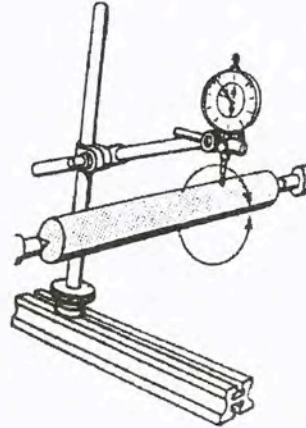
Σχήμα 3.2.3α. Μετρητικό ρολόι με τα εξαρτήματά του – Χρήση του μετρητικού ρολογιού για τον έλεγχο της κυλινδρικότητας άξονα
