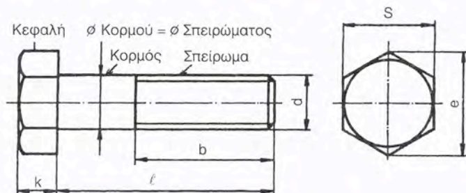
Σχήμα 7.1.1β Χαρακτηριστικές διαστάσεις ενός εξαγωνικού κοχλίου.
