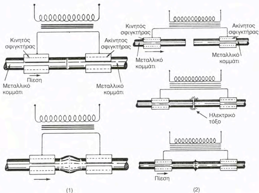
Σχήμα 8.4.12στ 1) Ηλεκτροσυγκόλληση αντιστάσεως κατά άκρα.
