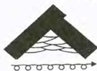
Σχήμα 8.4.86: Κινήσεις του ηλεκτροδίου για τη δημιουργία συγκόλλητικής ραφής στις διάφορες θέσης συγκόλλησης.
