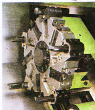
Σχήμα 1.3β: Σύγχρονος προγραμματιζόμενος τóρνος (CNC) και η εργαλειοφόρα κεφαλή του
