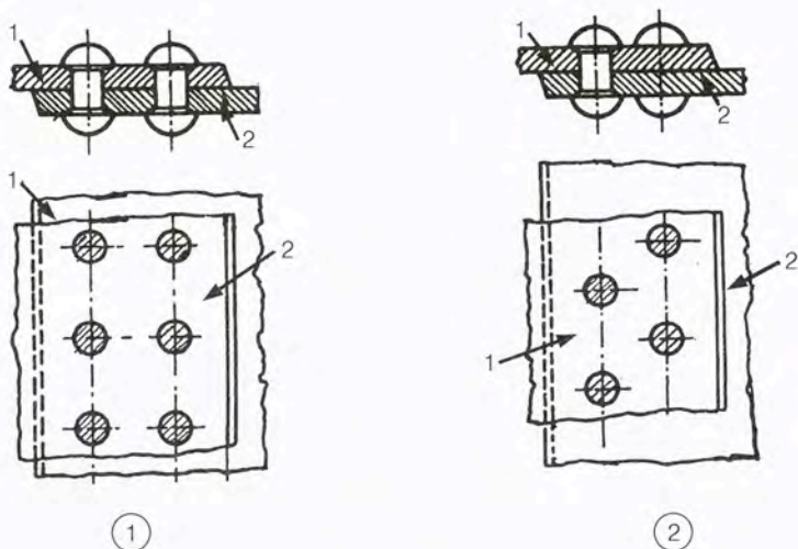
Σχήμα 7.1.2γ Ηλώσεις επικάλυψης: 1) Ηλώση διπλής σειράς καρφιών με διάταξη το ένα δίπλα στο άλλο. 2) Ηλώση διπλής σειράς καρφιών με διάταξη ζιγκ-ζαγκ.
