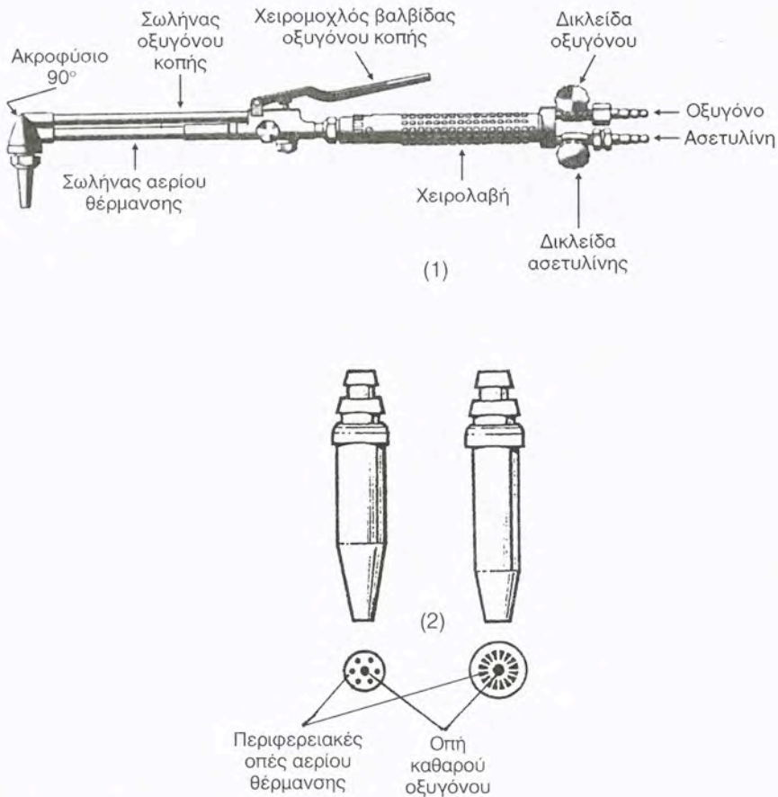
Σχήμα 8.3.126 1) Οξυγονοκόφτης. 2) Ακροφύσια οξυγονοκόφτη.
