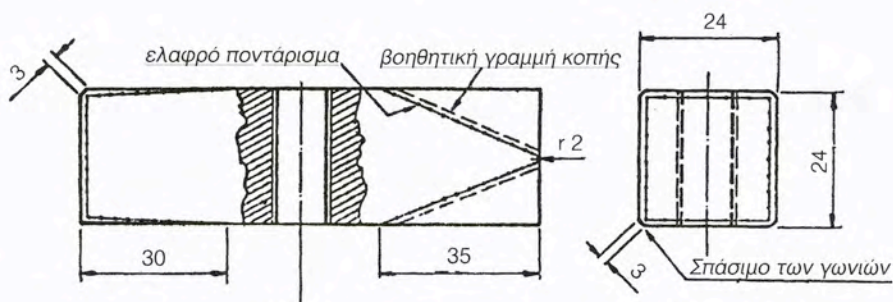
Πλάγια όψη
