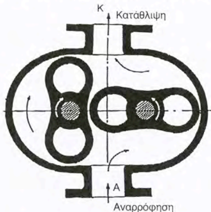
Σχήμα 16.1.1γ. Αντλία με περιστρεφόμενα έμβολα (λοβούς)
