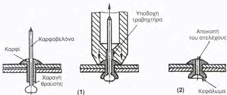
Σχήμα 7.1.20 Καρφωτή σύνδεση με χρήση τυφλοκαρφιού και κάρφωμα με μηχανικό τραβηχτήρα (πριτσίναδόρο).
