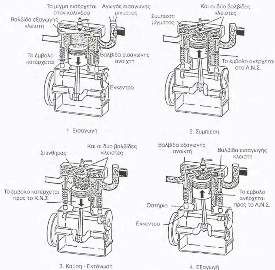
Σχήμα 14.2α Λειτουργία τετράχρονης βενζινομηχανής
