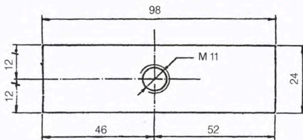
Κάτοψη
