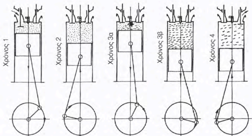
1. Εισαγωγή 2. Συμπίεση 3. Εγχυση - Καύση και εκτόνωση 4. Εξαγωγή
