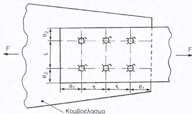
Σχήμα 7.1.1ε Αποστάσεις κοχλίων.
