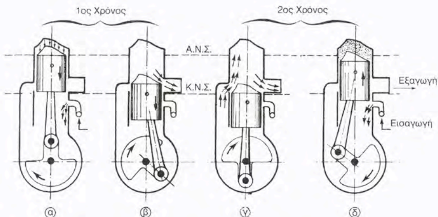
Σχήμα 14.2.1α Λειτουργία της δίχρονης βενζινομηχανής
