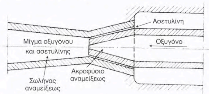
Σχήμα 8.3.7β: Τομή του καυστήρα χαμηλής πίεσεως στη θέση αναμειξεως των αερίων.
