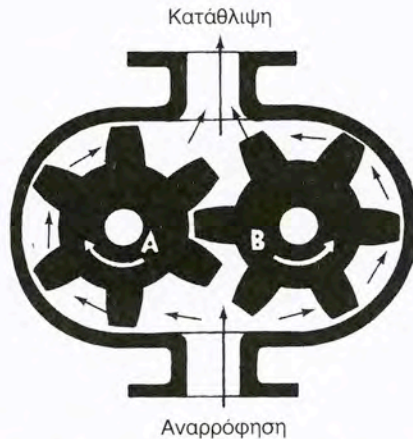
Σχήμα 16.1.1β. Αντλία με οδοντωτούς τροχούς Α: Κινητήριος οδοντωτός τροχός Β: Κινούμενος οδοντωτός τροχός
