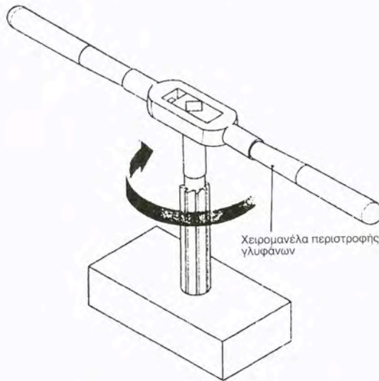
Σχήμα 4.15γ. Γλύφανση τρύπας
