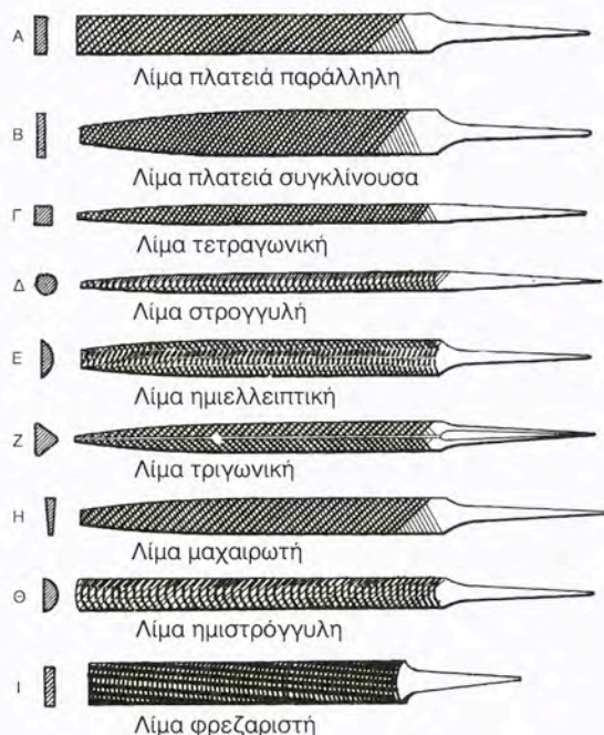
Σχήμα 4.126. Είδη λιμών
