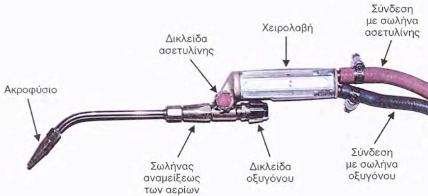
Σχήμα 8.3.7α: Καυστήρας οξυγονοσυγκόλλησης.
