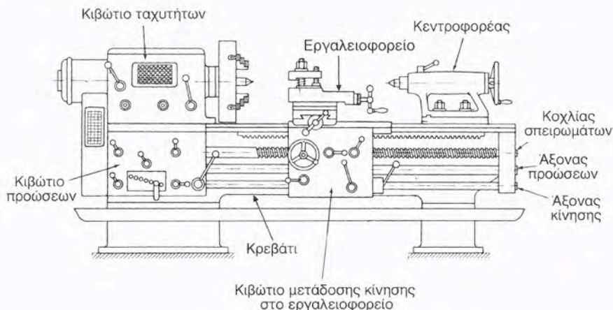
Σχήμα 13.2α. Τα κύρια μέρη του τόρνου
