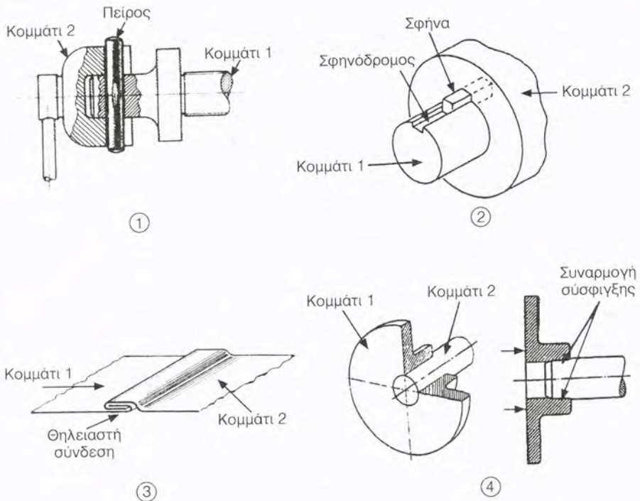
Σχήμα 7.16 1) Σύνδεση με πείρο, 2) Σφηνοσύνδεση, 3) Θηλειαστή σύνδεση, 4) Σύνδεση με συναρμογή σύσφιγξης (σφικτή σύνδεση).
