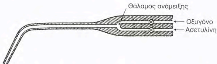
Σχήμα 8.3.7γ: Τομή του καυστήρα υψηλής πίεσεως στη θέση αναμείξεως των αερίων.
