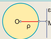
εξωτερική
