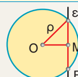
τέμνουσα
