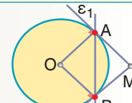
εφαπτόμενα τμήματα
