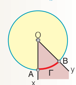
επίκεντρη γωνία
