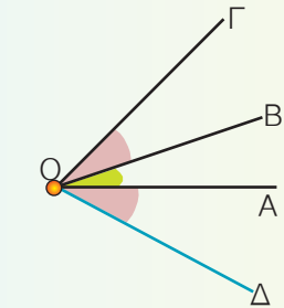
διαδοχικές γωνίες
