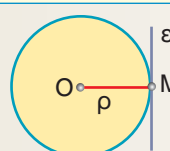
εφαπτόμενη
