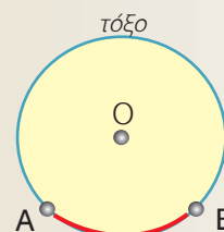
τόξο
