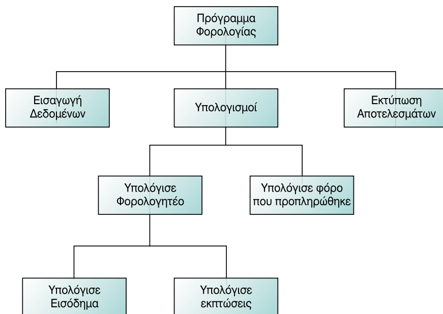
Σχ. 6.4. Ιεραρχική σχεδίαση υπολογισμού του φόρου εισοδήματος
