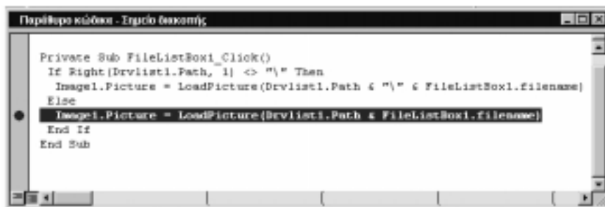
Σχ. 13.2. Σημείο διακοπής στον κώδικα της εφαρμογής
