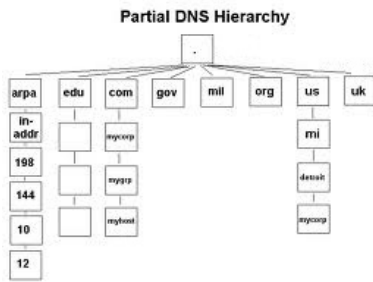
Εικόνα 9.3. Ιεραρχία DNS
