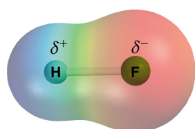
Κατανομή ηλεκτρικού φορτίου στο μόριο του \text{HF} .
