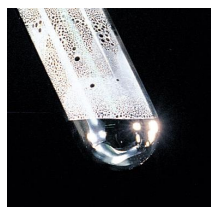
Με θέρμανση το οξείδιο του υδραργύρου (II), \text{HgO} , διασπάται παράγοντας \text{Hg(l)} και \text{O}_2 .
