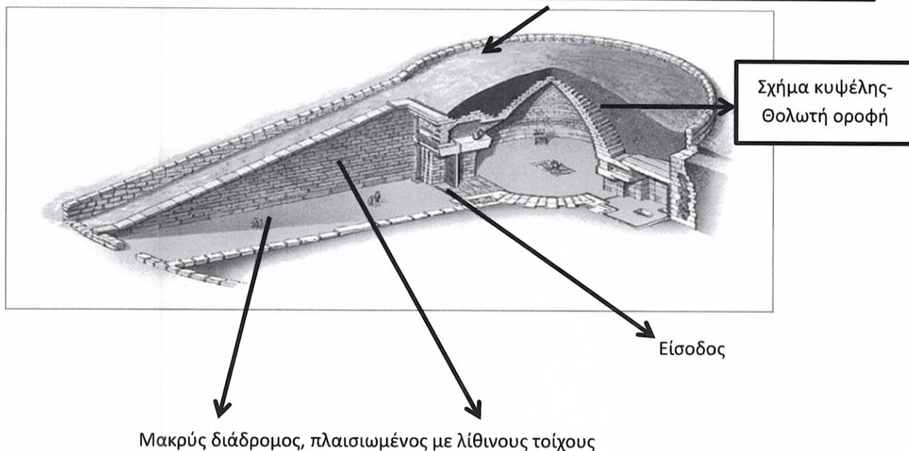
Εικόνα 2: Σχεδιαστική τομή του Θησαυρού του Ατρέως (πηγή εικόνας –χωρίς επεξηγήσεις: http://www.hellinon.net/ANEOMENA/TholotoiTafoi.htm )
