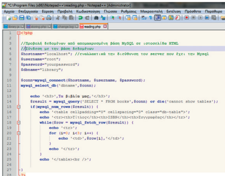
Σχήμα 5.23: Προβολή δεδομένων σε HTML από MySQL
