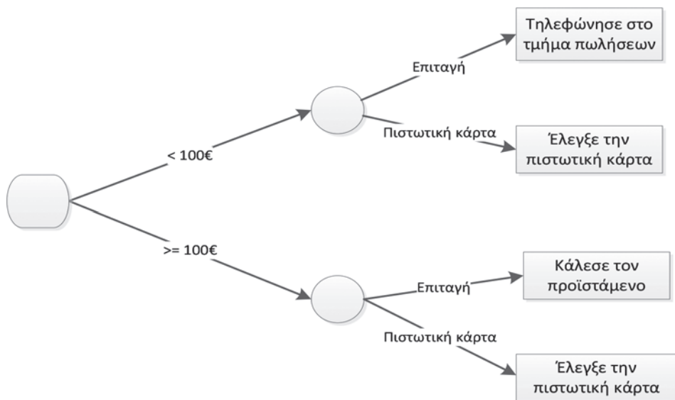
Σχήμα 3.10: Δένδρο αποφάσεων
