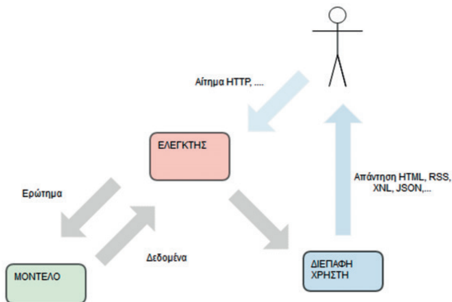
Σχήμα 5.25: Ένα βασικό MVC αίτημα
