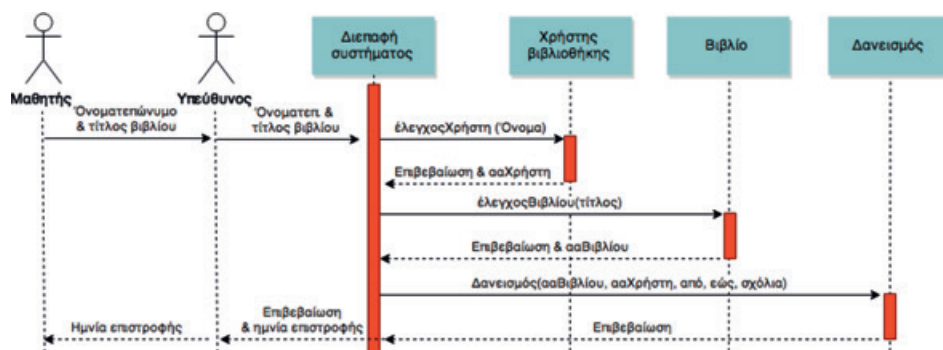
Σχήμα 4.13: Διάγραμμα ακολουθίας δανεισμού
