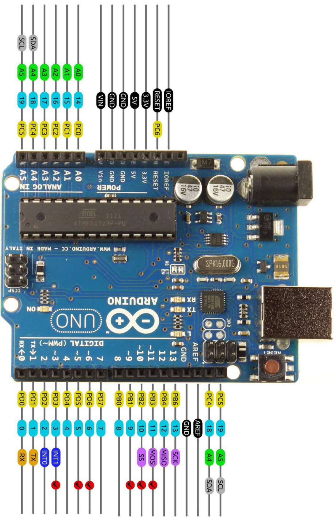
Εικόνα 4 : Οι ακίδες του Arduino Uno R3
