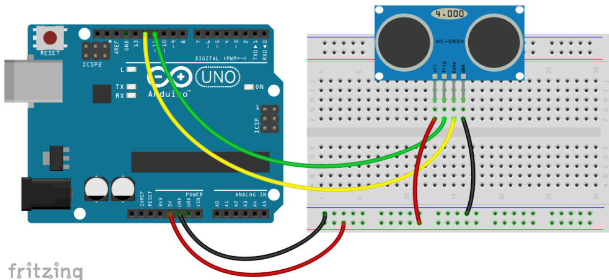
Εικόνα 60: Σύνδεση του αισθητήρα υπερήχων στον Arduino
