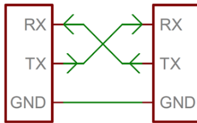
Εικόνα 71: Σειριακή σύνδεση δύο συσκευών
