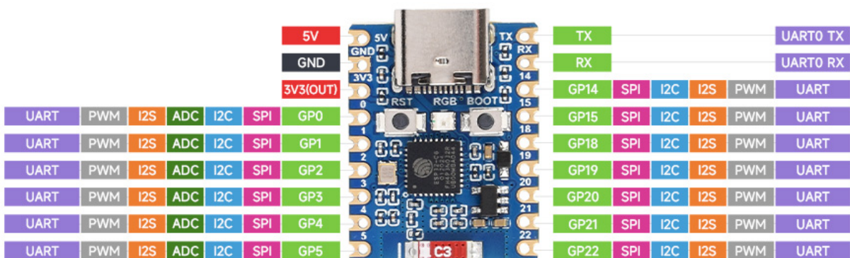
Εικόνα 96: Πλακέτα με τον ESP32-C6
