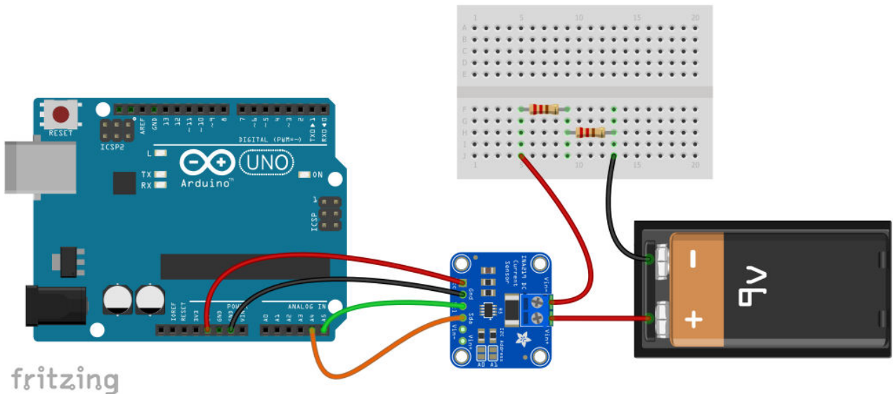
Εικόνα 64: Σύνδεση μονάδας INA219 στον Arduino για μέτρηση ρεύματος
