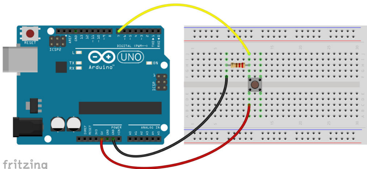
Εικόνα 18: Σύνδεση διακόπτη push button στον Arduino
