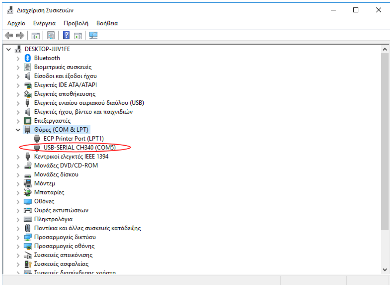
Εικόνα 14: Διαχείριση συσκευών - στη θύρα COM5 ο υπολογιστής "συνομιλεί" με τον Arduino (CH-340 κλώνο)
