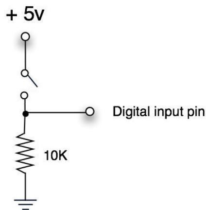
Εικόνα 17: Σχηματικό διάγραμμα σύνδεσης διακόπτη στον Arduino
