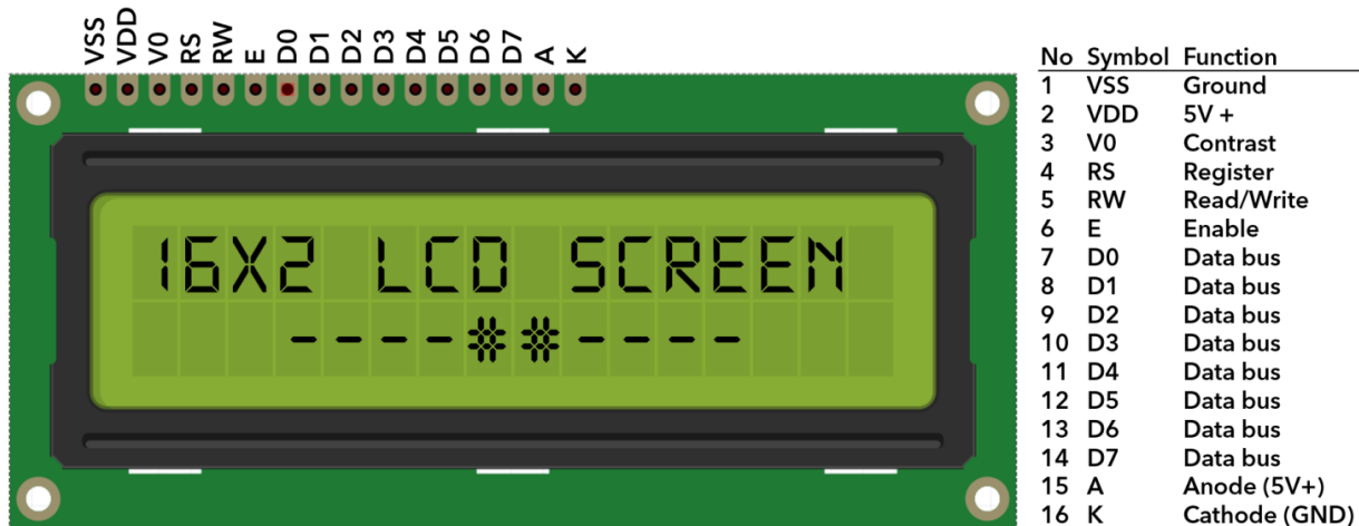
Εικόνα 35: LCD παράλληλης διεπαφής
