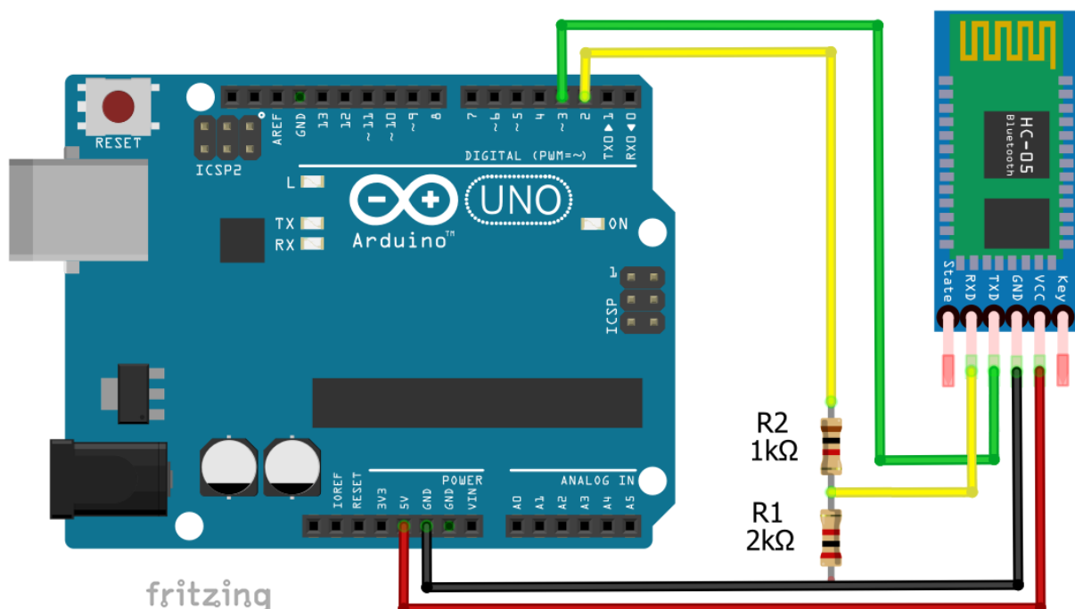
Εικόνα 70: Σύνδεση της μονάδας HC-05 στον Arduino (αντίστοιχες είναι και οι συνδέσεις της μονάδας HC-06)
