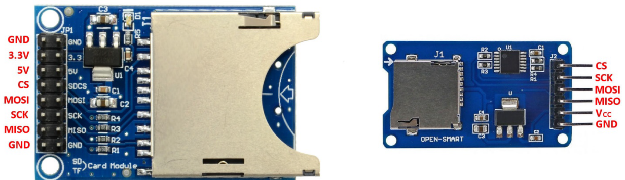
Εικόνα 45 : Αριστερά η μονάδα SD Card και δεξιά η μονάδα micro SD Card
