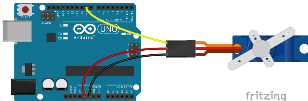
Εικόνα 25 : Σύνδεση σερβοκινητήρα στον Arduino
