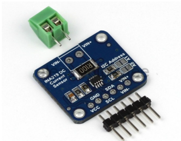
Εικόνα 63: Προσυναρμολογημένη μονάδα INA219
