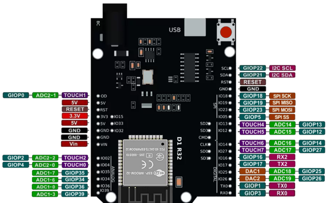
Εικόνα 93: Wemos D1 R32 v1.0.0
