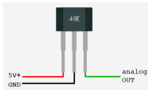
Εικόνα 49: Ο αναλογικός αισθητήρας μαγνητικού πεδίου
