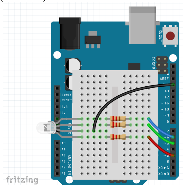
Εικόνα 88: Σύνδεση ενός RGB LED κοινής καθόδου στον Arduino
