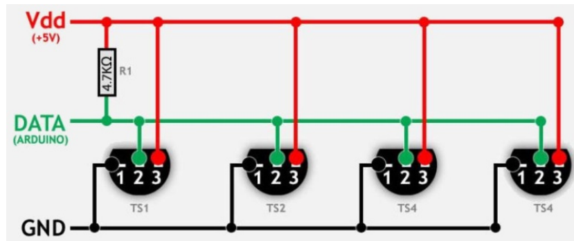
Εικόνα 40: Αισθητήρες DS18B20 σε κανονικό τρόπο λειτουργίας
