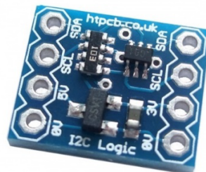
Εικόνα 31: Μονάδα αμφίδρομης μετατόπισης επιπέδου τάσης
