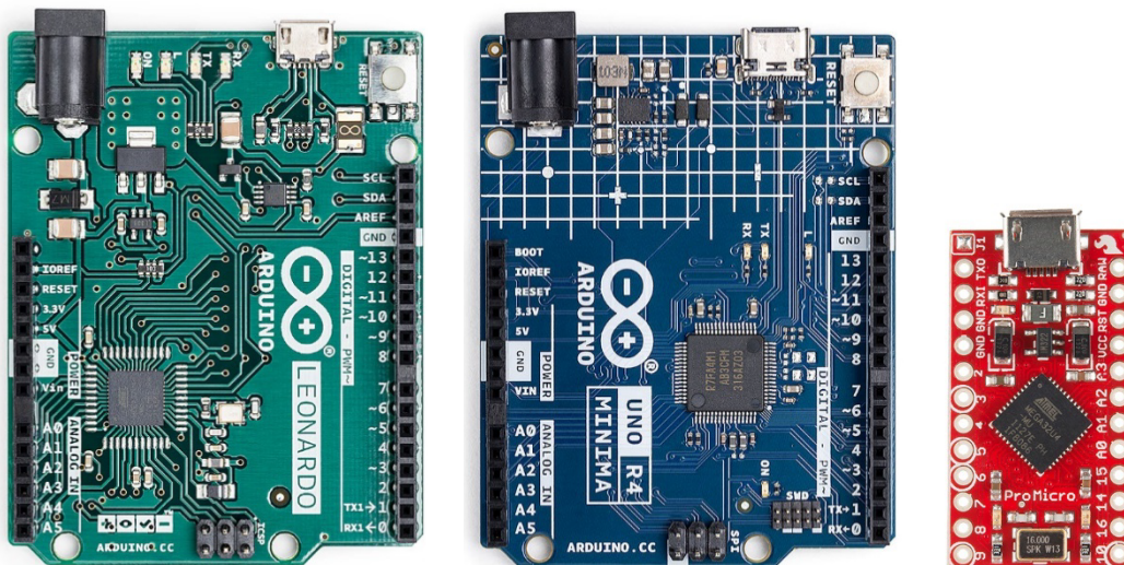
Εικόνα 8: Από αριστερά: Arduino Leonardo, Arduino Uno R4 Minima και Sparkfun Arduino Micro
