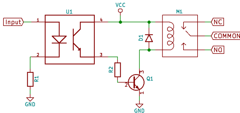
Εικόνα 53: Το κυκλωματικό διάγραμμα της μονάδας ρελέ
