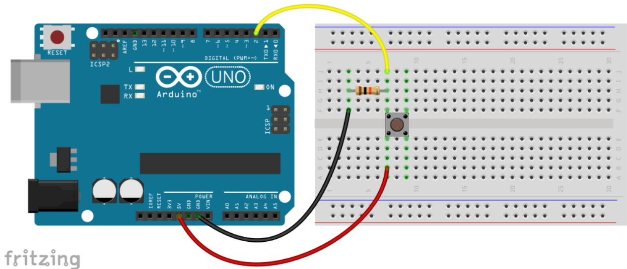
Εικόνα 48: Σύνδεση διακόπτη στην ψηφιακή είσοδο 2 του Arduino
