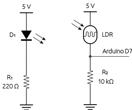
Εικόνα 82: Το κυκλωματικό διάγραμμα μιας απλής φωτοπύλης για χρήση με τον Arduino
