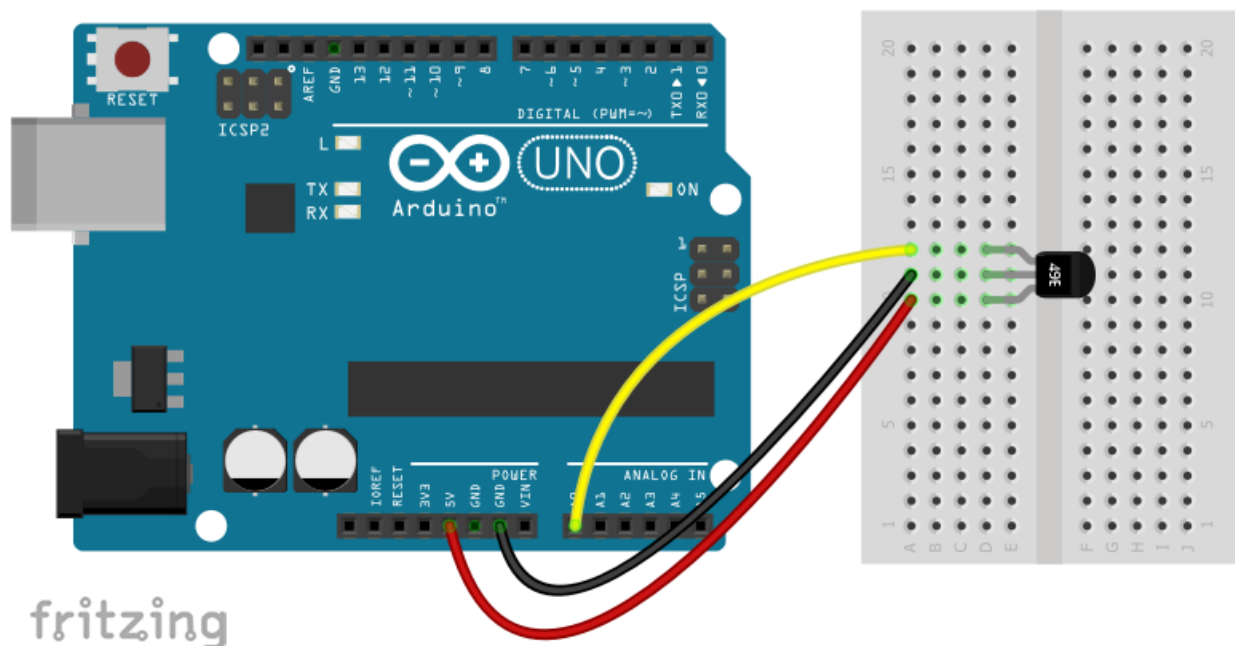
Εικόνα 50: Σύνδεση αισθητήρα μαγνητικού πεδίου στον Arduino
