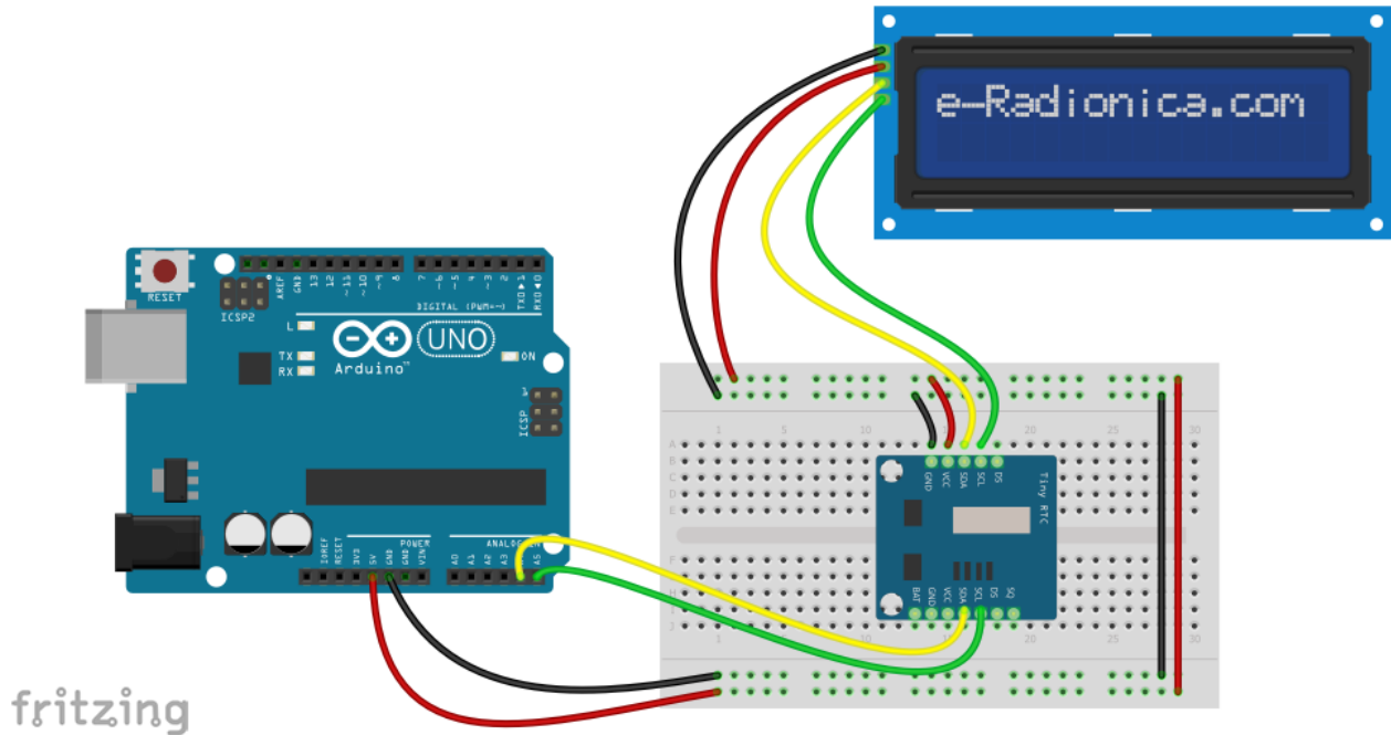
Εικόνα 62: Ρολόι πραγματικού χρόνου με οθόνη υγρών κρυστάλλων
