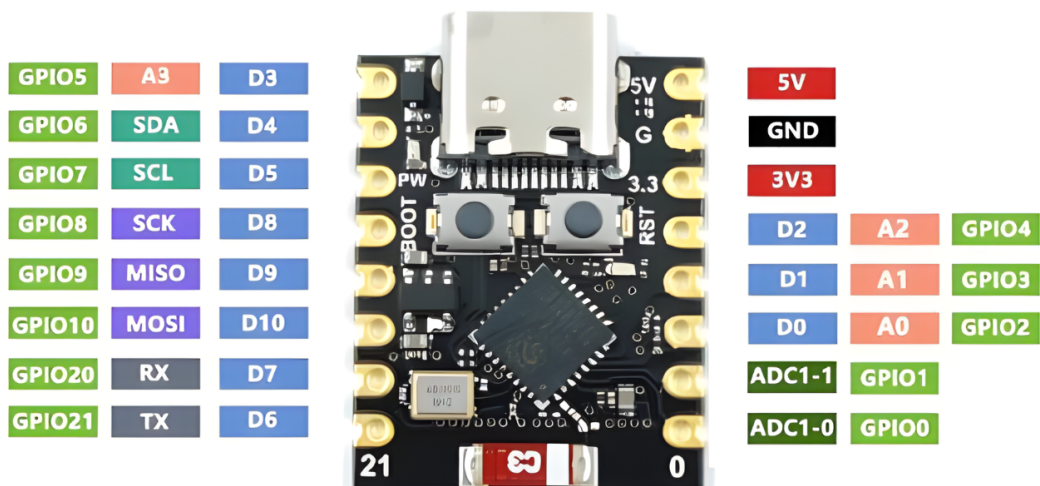
Εικόνα 95: Πλακέτα με τον ESP32-C3
