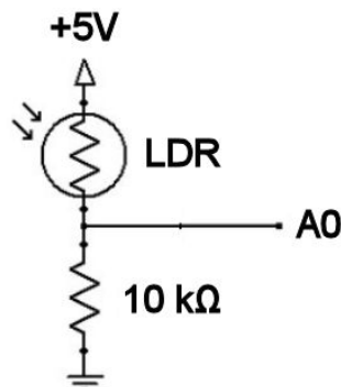
Εικόνα 22: Διαιρέτης τάσης με φωτοαντίσταση
