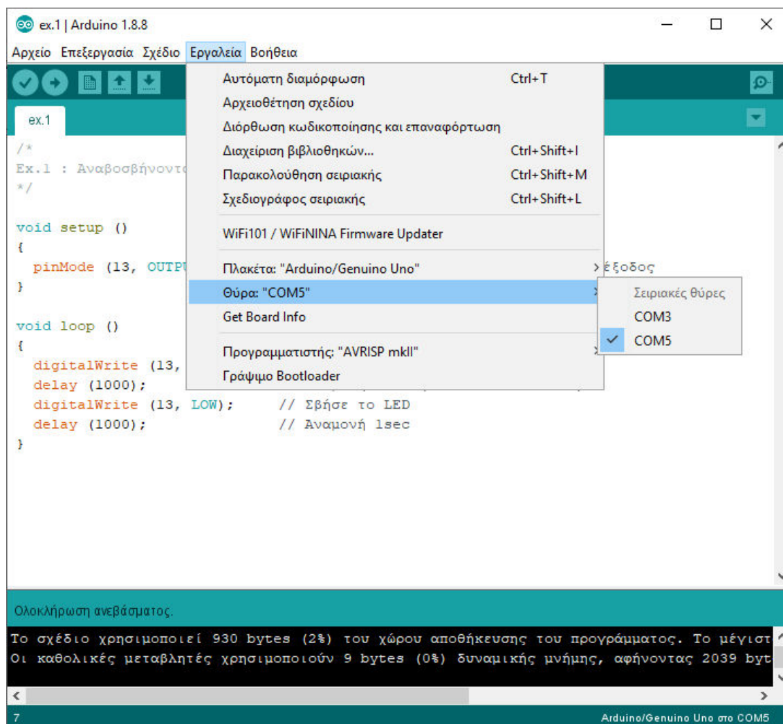
Εικόνα 13 : Επιλογή σειριακής θύρας
