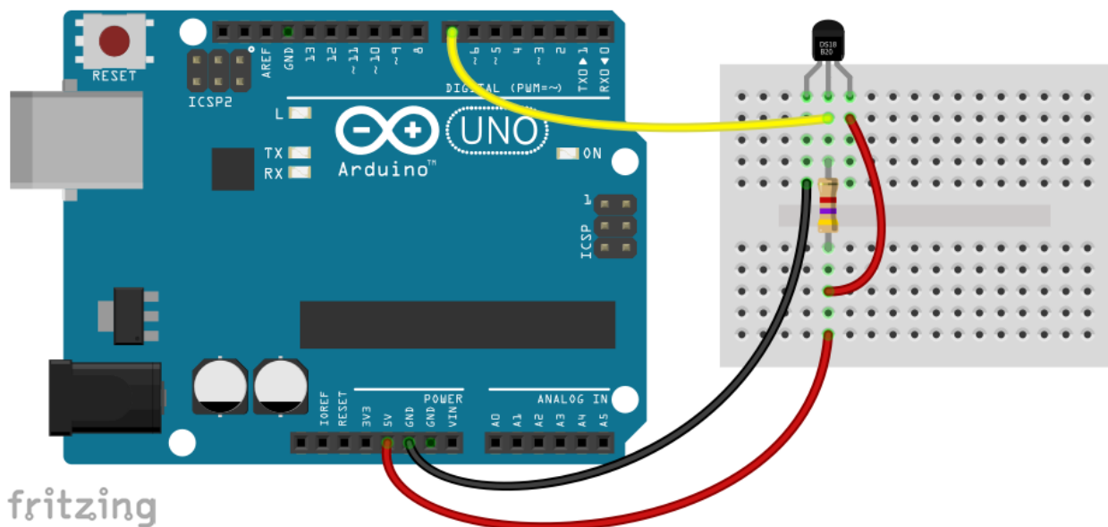
Εικόνα 42: Σύνδεση του αισθητήρα DS18B20 στον Arduino
