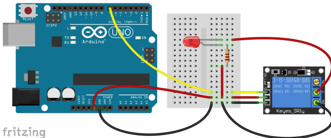
Εικόνα 55: Σύνδεση της μονάδας ρελέ στον Arduino
