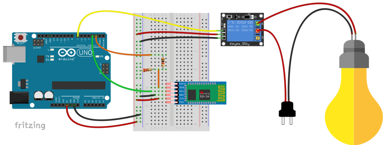
Εικόνα 81: Το κύκλωμα του αυτοματισμού
