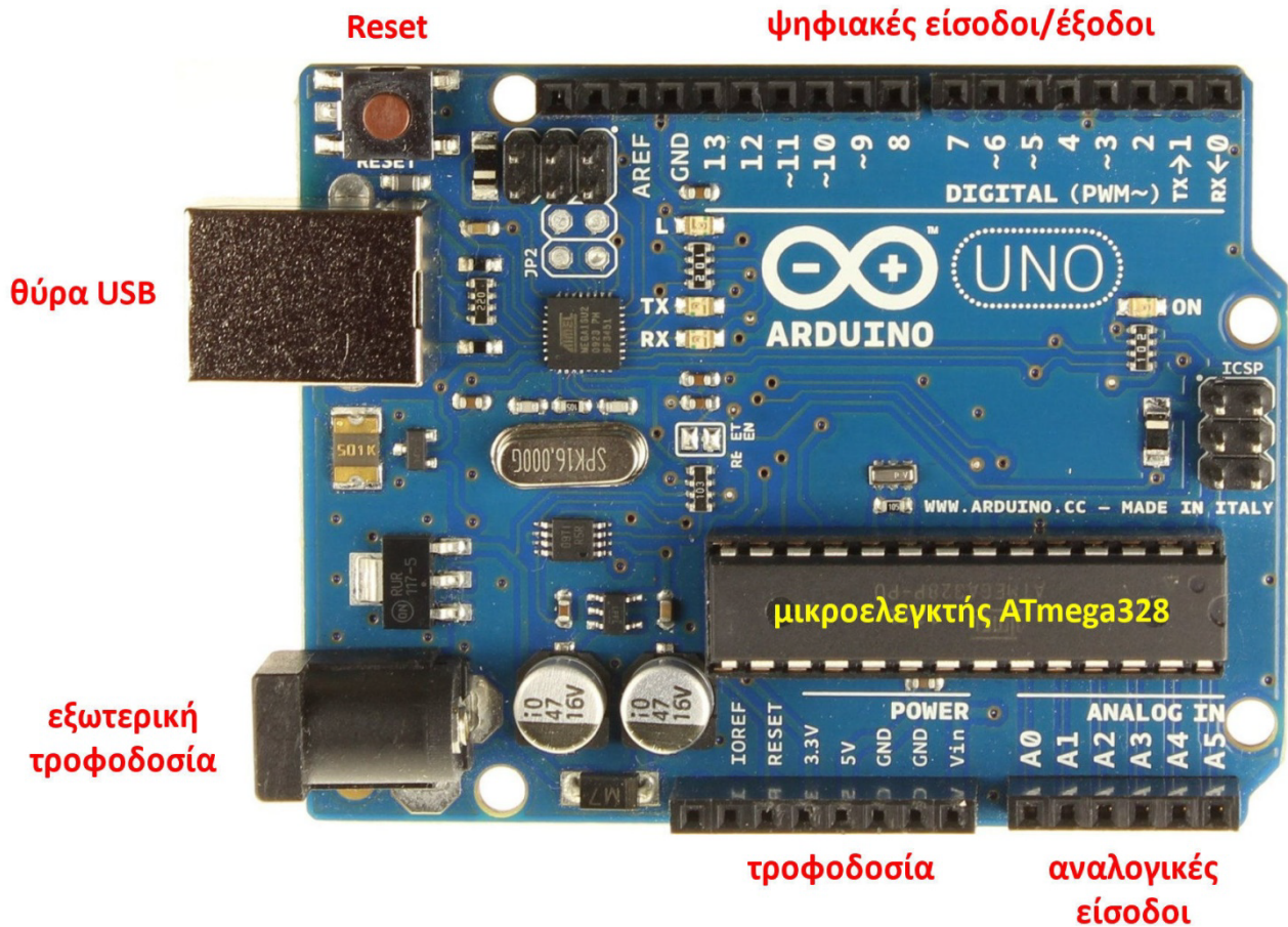
Εικόνα 2: Η πλακέτα του Arduino Uno R3
