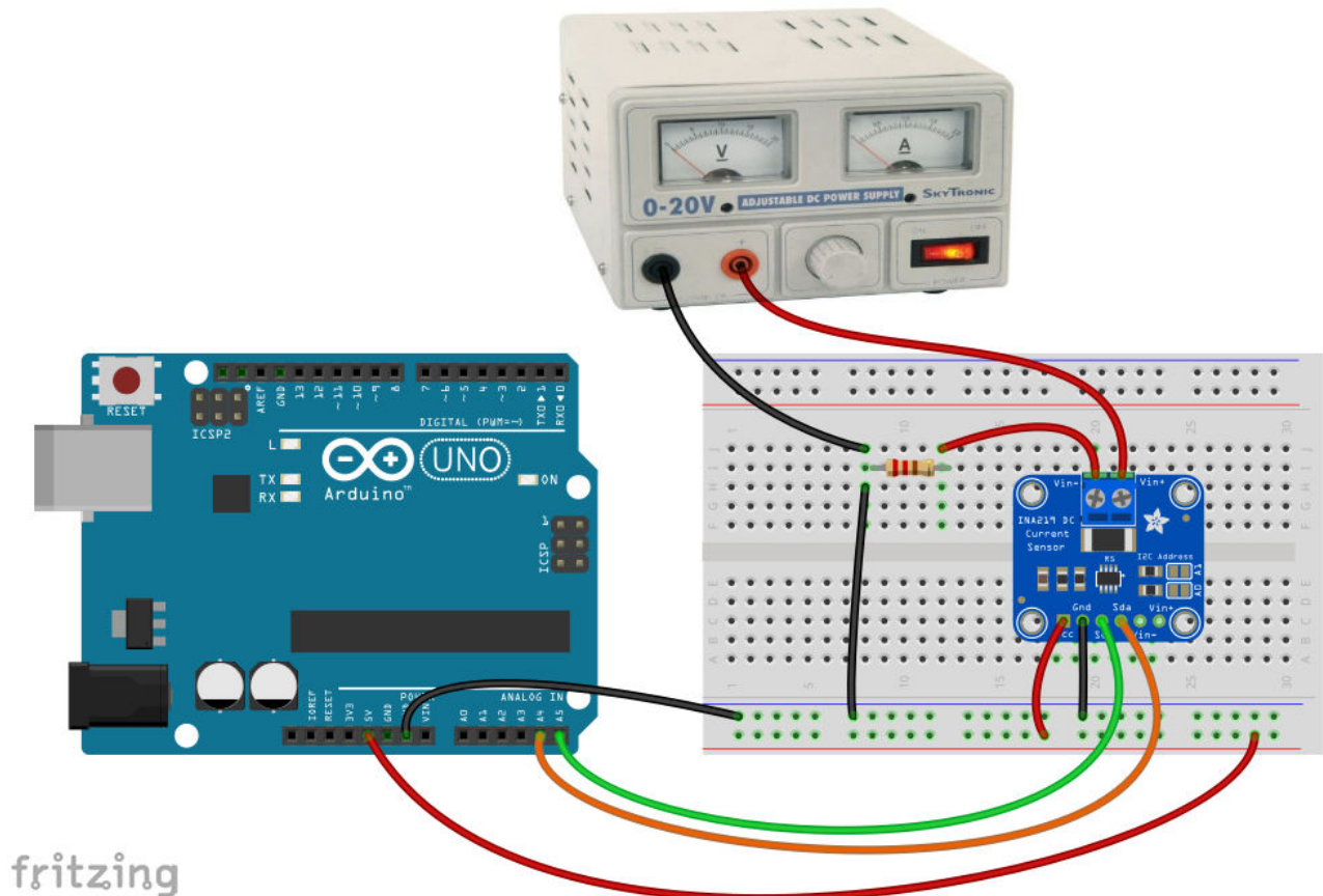
Εικόνα 66: Συνδεσμολογία για το πείραμα του νόμου του Ohm
