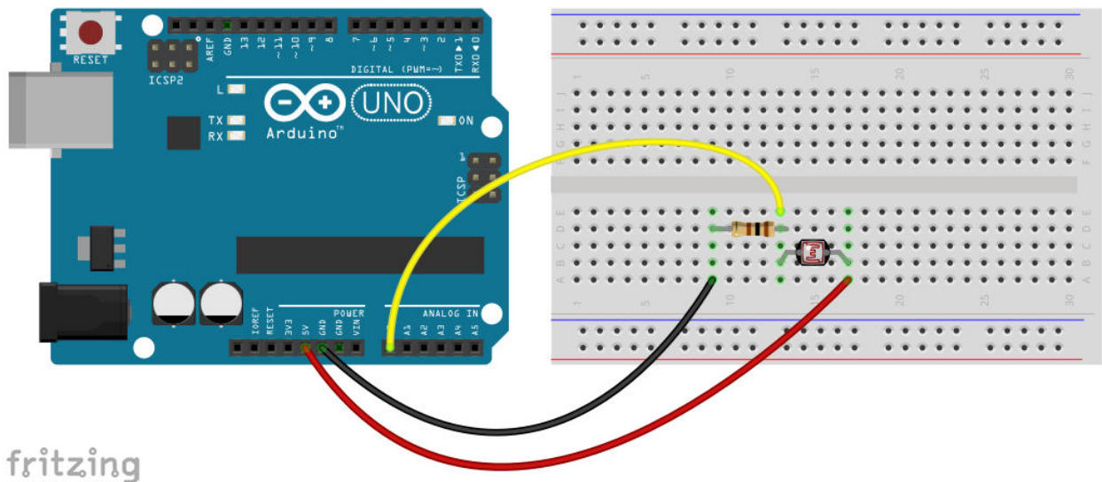
Εικόνα 23: Σύνδεση φωτοαντίστασης στον Arduino
