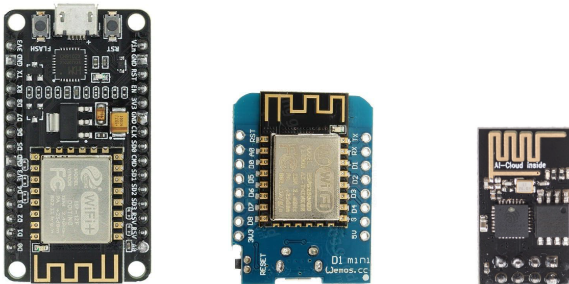
Εικόνα 91: Συστήματα ESP8266. Από αριστερά: NodeMCU, Wemos D1 mini και η μονάδα ESP-01
