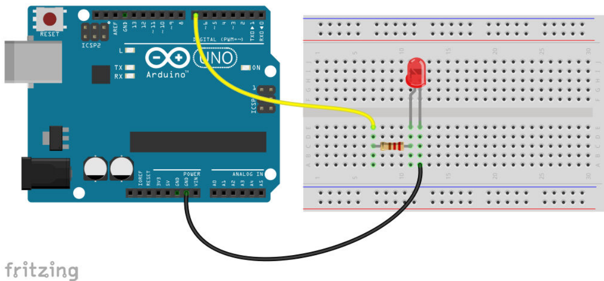
Εικόνα 16: Σύνδεση LED στον Arduino
