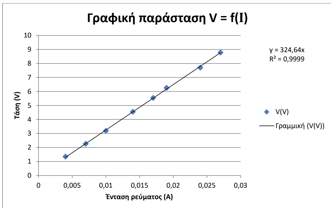
Εικόνα 68 : Η γραφική παράσταση V = f(I)
