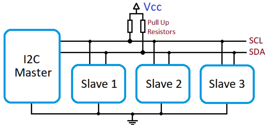
Εικόνα 28: Ο δίαυλος I 2 C
