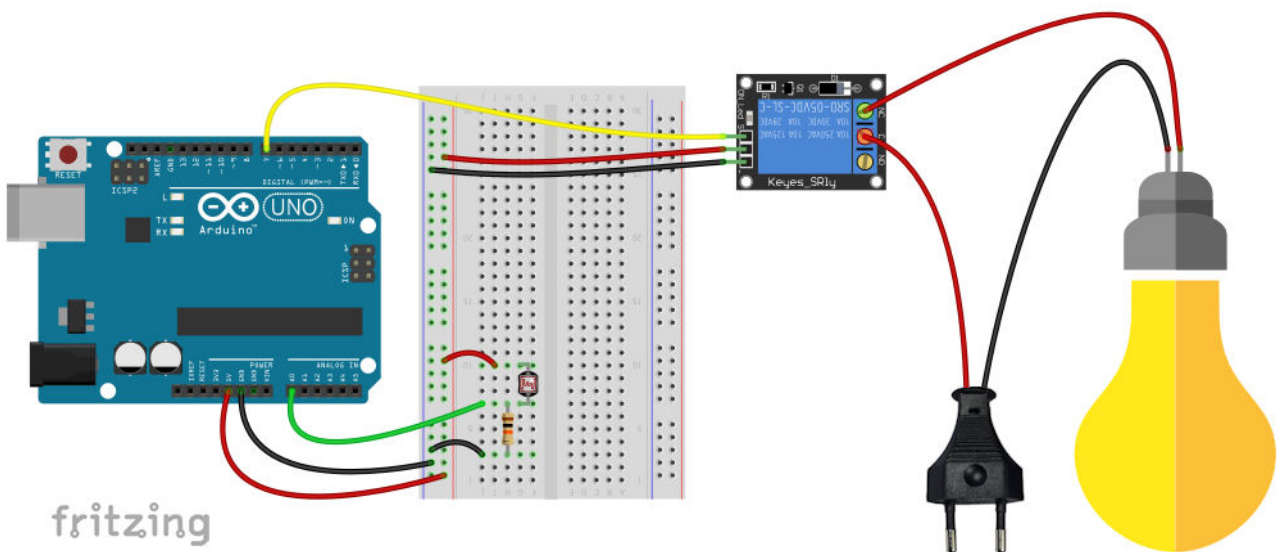
Εικόνα 57: Κύκλωμα απλού αυτοματισμού με λάμπα 220 V
