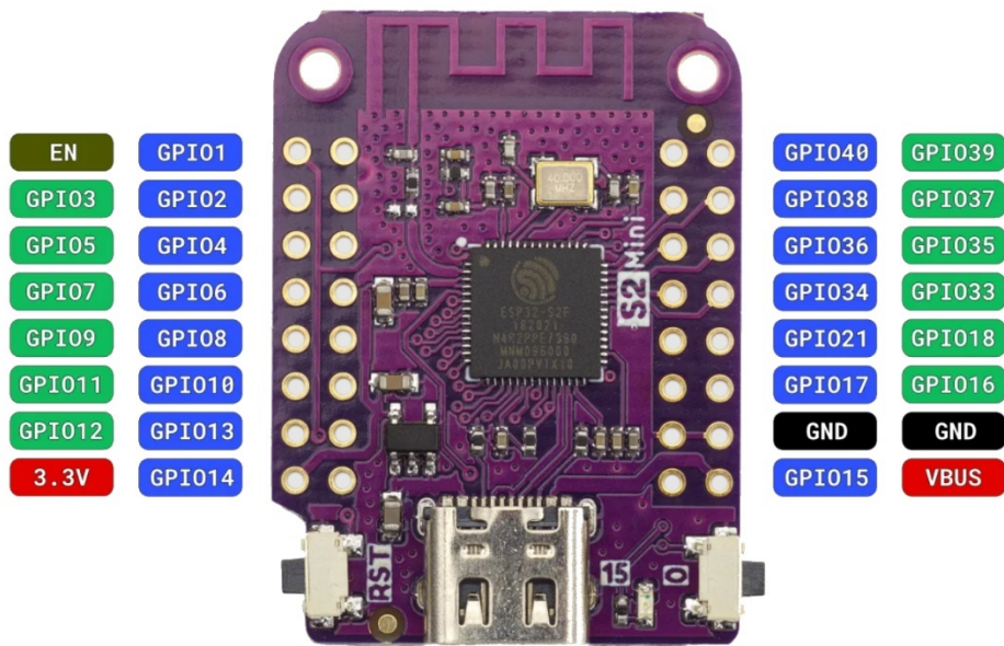
Εικόνα 94: Πλακέτα με τον ESP32-S2
