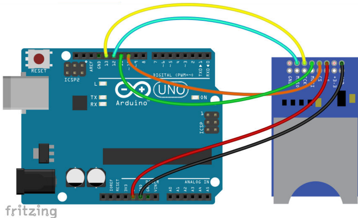
Εικόνα 47 : Σύνδεση της μονάδας SD Card στον Arduino
