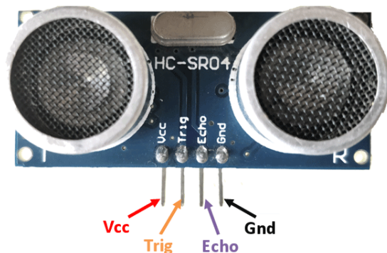
Εικόνα 58: Ο αισθητήρας υπερήχων HC-SR04
