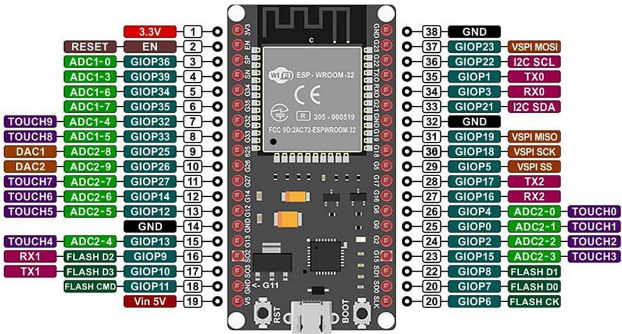
Εικόνα 92: ESP32 DEVKIT v1
