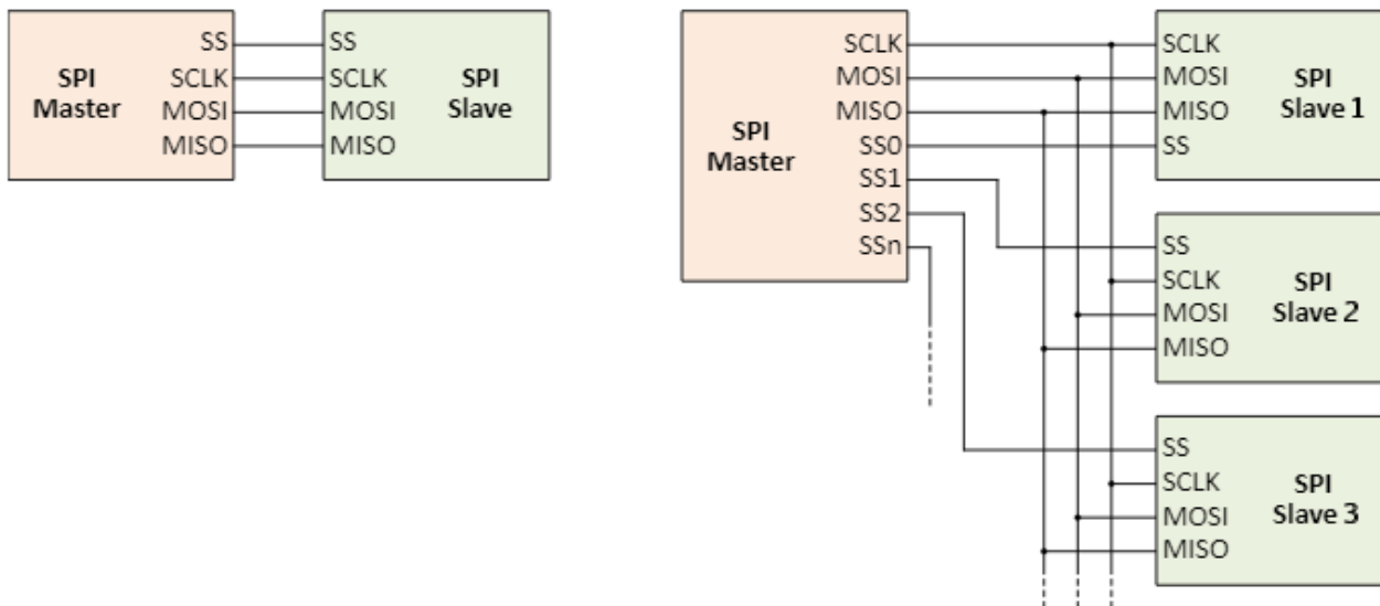
Εικόνα 44: Σύνδεση στο δίαυλο SPI
