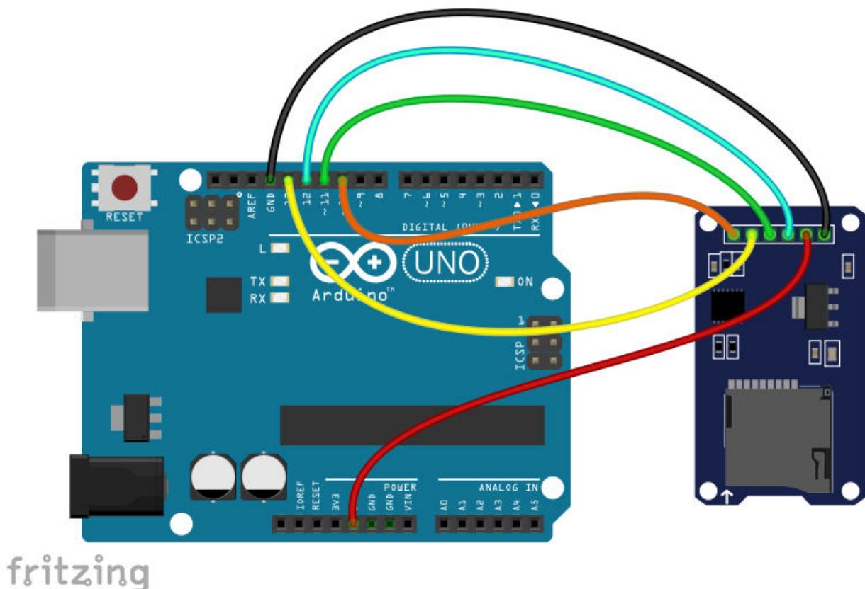
Εικόνα 46: Σύνδεση μονάδας κάρτας micro SD στον Arduino
