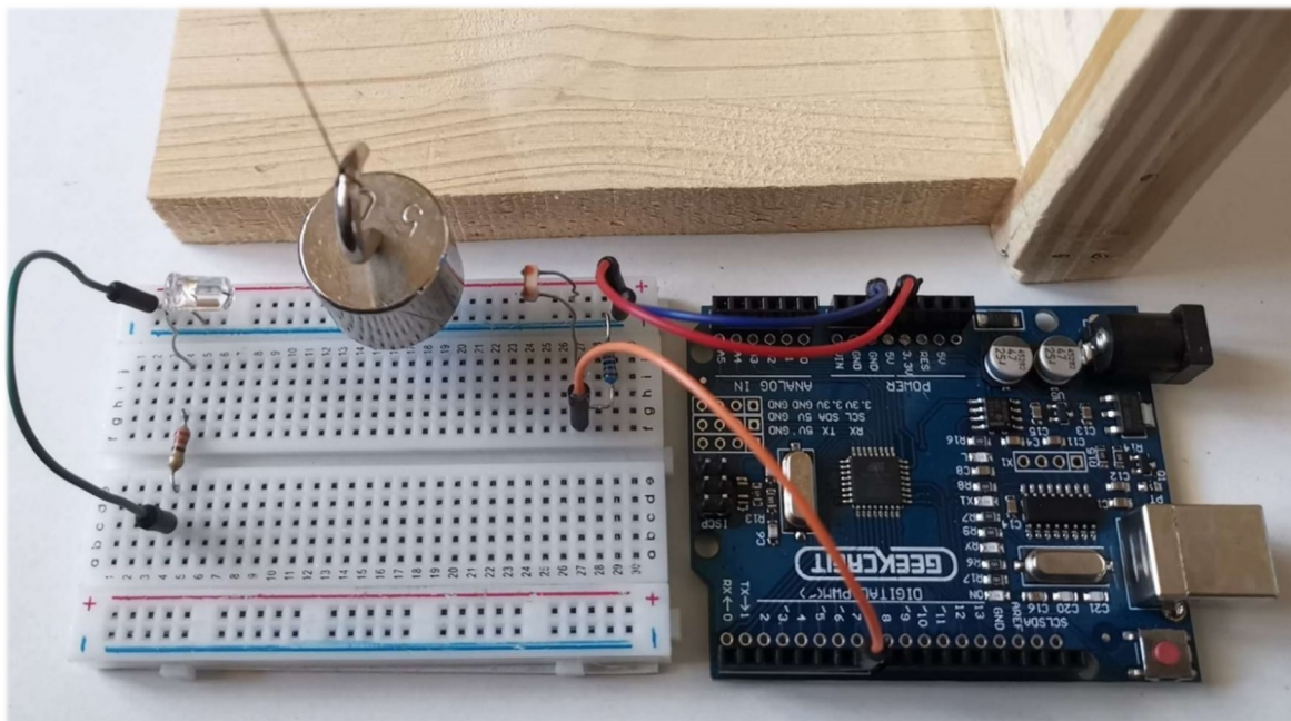
Εικόνα 85: Λεπτομέρεια της πειραματικής διάταξης για τη μέτρηση της περιόδου εκκρεμούς
