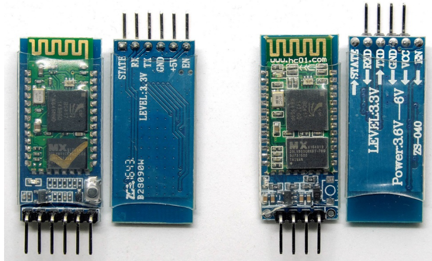
Εικόνα 69: Οι μονάδες HC-05 (αριστερά) και HC-06 (δεξιά)
