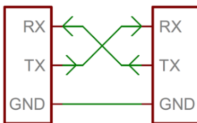
Εικόνα 19: Σειριακή σύνδεση δύο συσκευών
