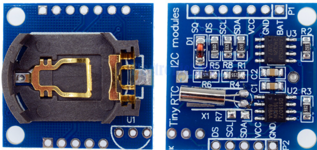
Εικόνα 33: Η μονάδα RTC DS1307 (Tiny RTC)
