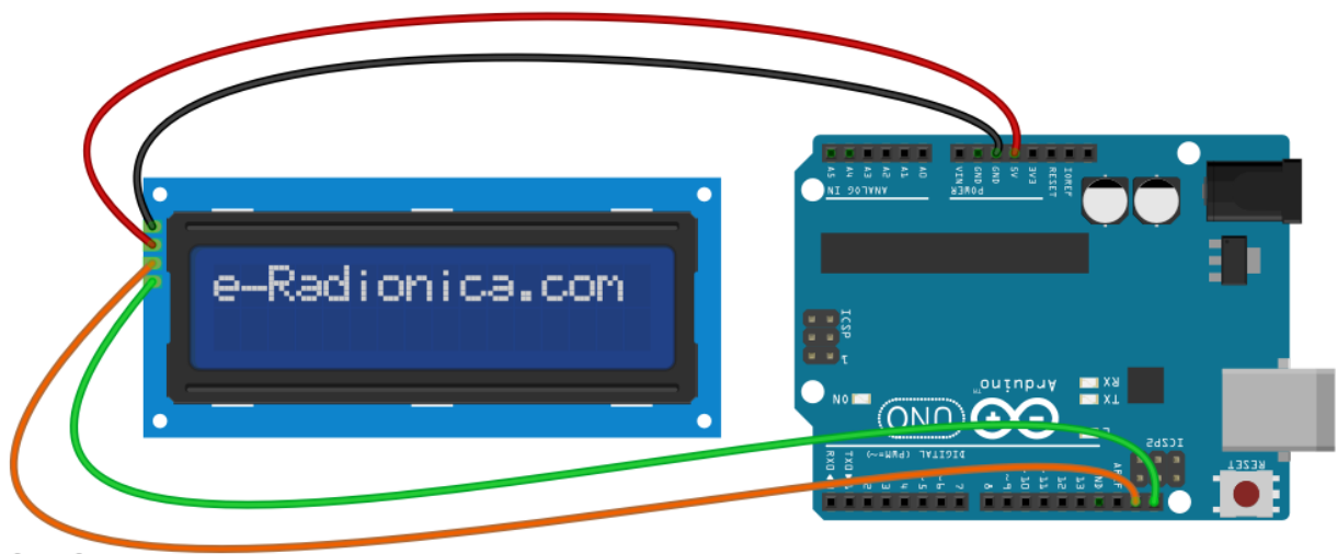
Εικόνα 37: Σύνδεση του LCD στον Arduino
