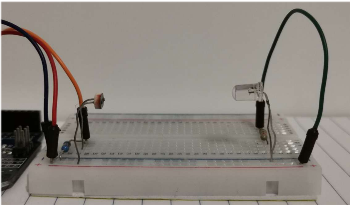
Εικόνα 84: Κατασκευή του πρωτοτύπου της φωτοπύλης
