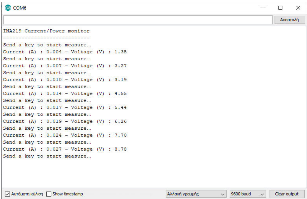
Εικόνα 67 : Πειραματικά δεδομένα για την επιβεβαίωση του Νόμου του Ohm
