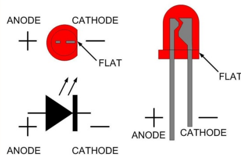
Εικόνα 15: Η δίοδος εκπομπής φωτός (LED)
