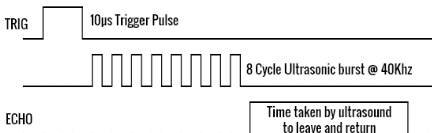
Εικόνα 59: Κύκλος λειτουργίας του αισθητήρα HC-SR04
