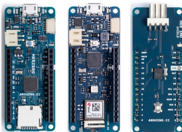
Εικόνα 7: Πλακέτες της οικογένειας MKR. Από αριστερά: MKR Zero, MKR WiFi 1010, MKR IMU Shield
