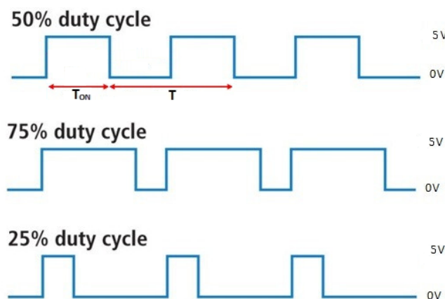
Εικόνα 90: Παλμοί διαφορετικού κύκλου εργασίας
