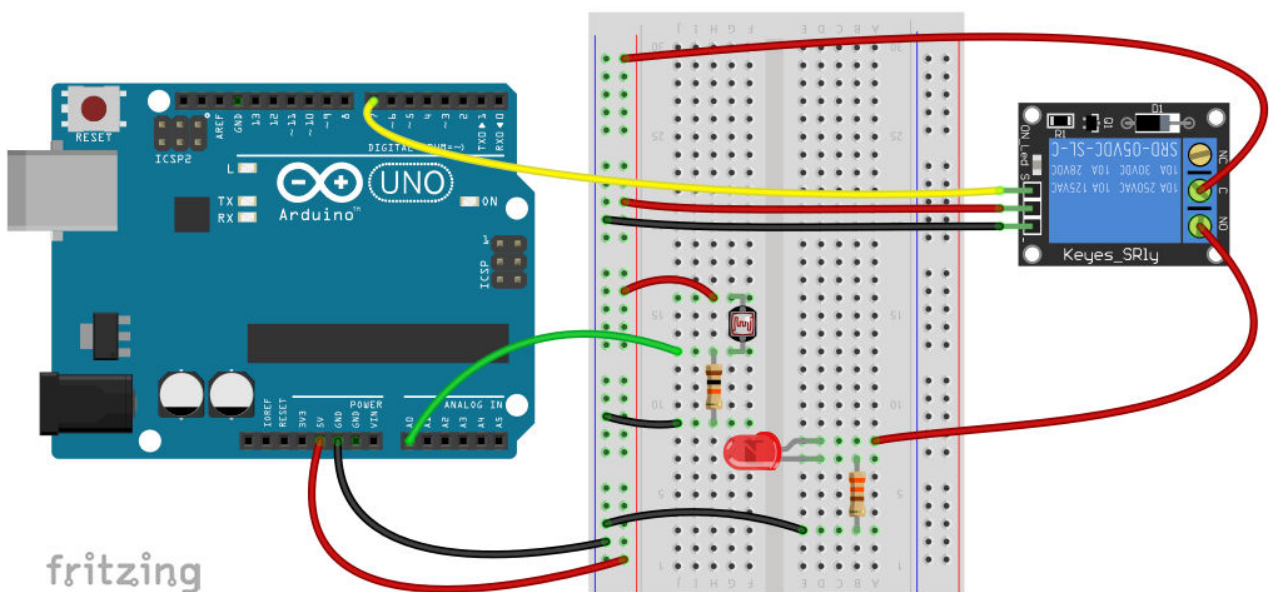
Εικόνα 56: Σύνδεση ρελέ, LED και φωτοαντίστασης στον Arduino
