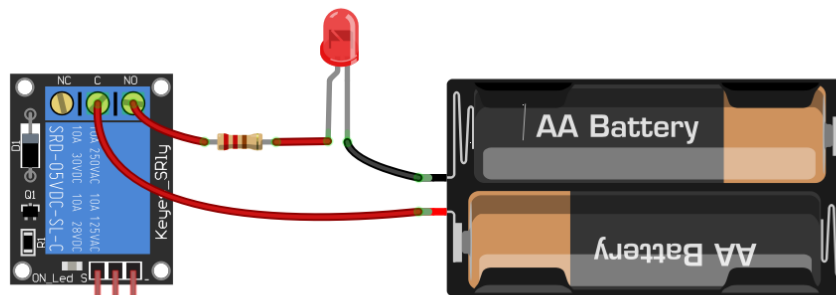
Εικόνα 54: Το ρελέ ως διακόπτης
