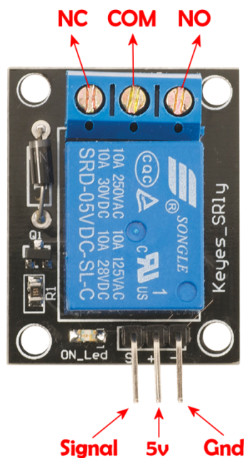
Εικόνα 52: Η μονάδα ρελέ
