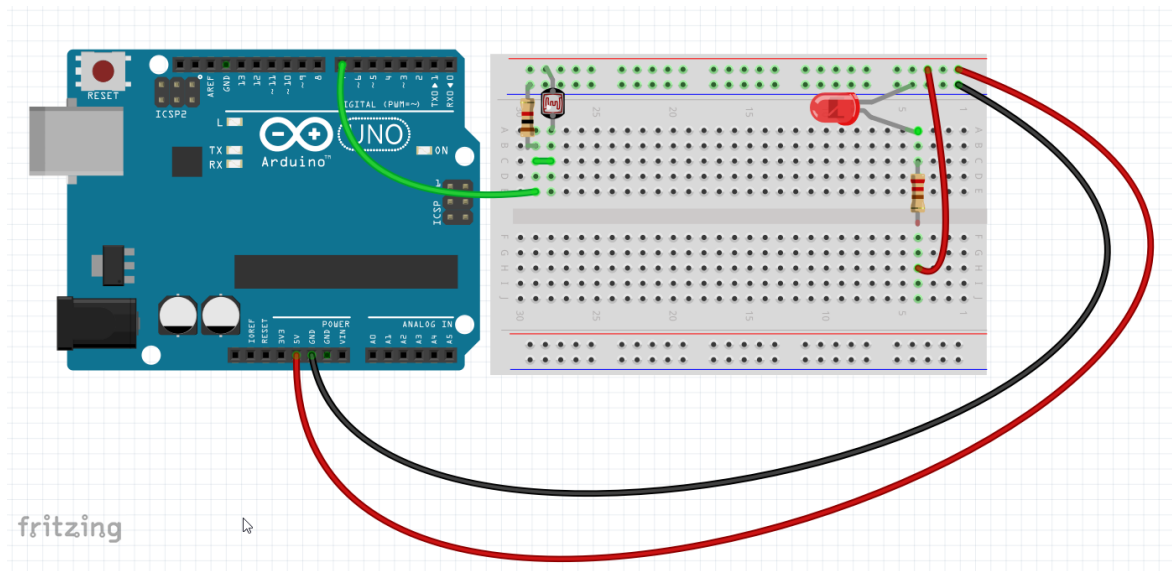
Εικόνα 83: Η φωτοπύλη σε breadboard
