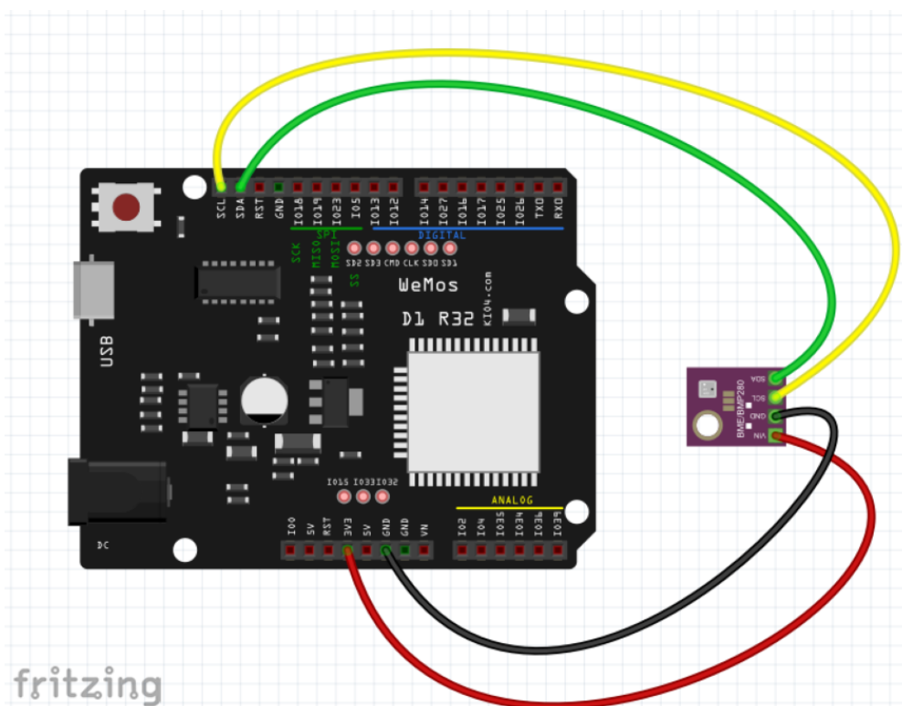
Εικόνα 99: Σύνδεση μονάδας BME280 στον Wemos D1 R32
