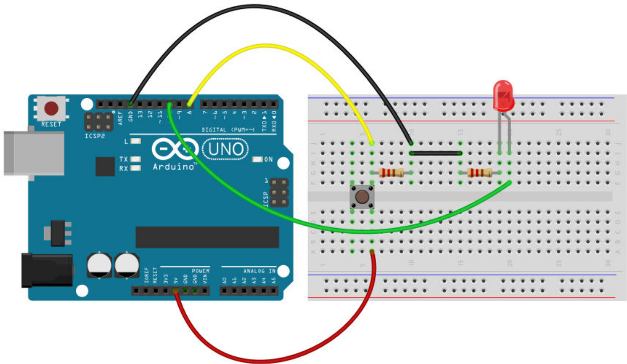
Εικόνα 21: LED και διακόπτης push button στον Arduino
