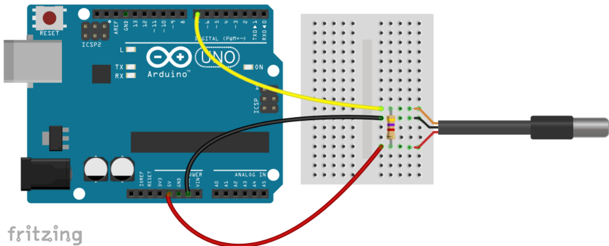
Εικόνα 43: Σύνδεση της αδιάβροχης εκδοχής του DS18B20 στον Arduino
