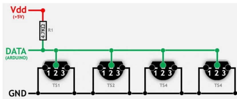
Εικόνα 41: Αισθητήρες DS18B20 σε παρασιτικό τρόπο λειτουργίας
