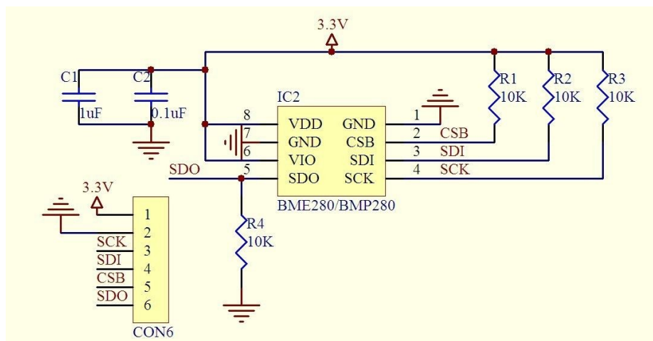
Εικόνα 30: Το σχηματικό διάγραμμα του αισθητήρα BMP280
