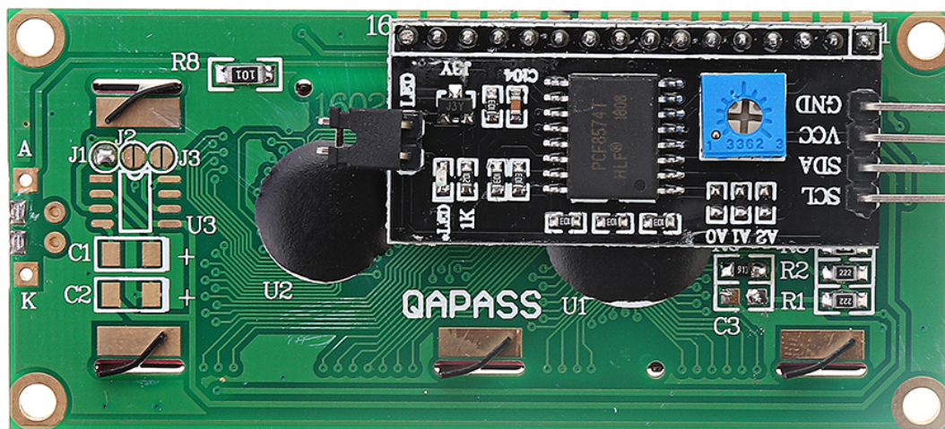
Εικόνα 36: Οθόνη LCD με I 2 C διεπαφή (πίσω όψη)
