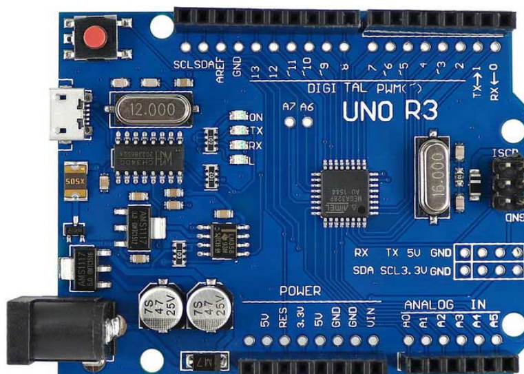
Εικόνα 3: Arduino Uno R3 κλώνος
