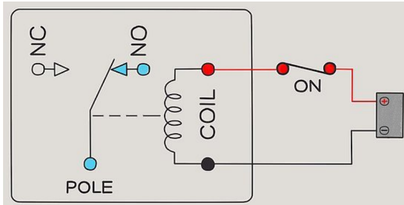
Εικόνα 51: Ο ηλεκτρονόμος ή ρελέ (relay)
