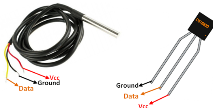
Εικόνα 39: Ο αισθητήρας DS18B20 (αδιάβροχη μορφή και μορφή ολοκληρωμένου 3 ακιδών)
