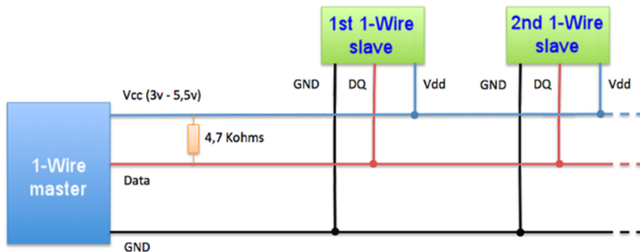
Εικόνα 38: Ο δίαυλος 1-Wire
