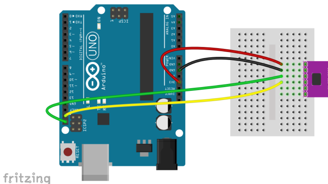
Εικόνα 32: Σύνδεση της μονάδας BMP280 στον Arduino
